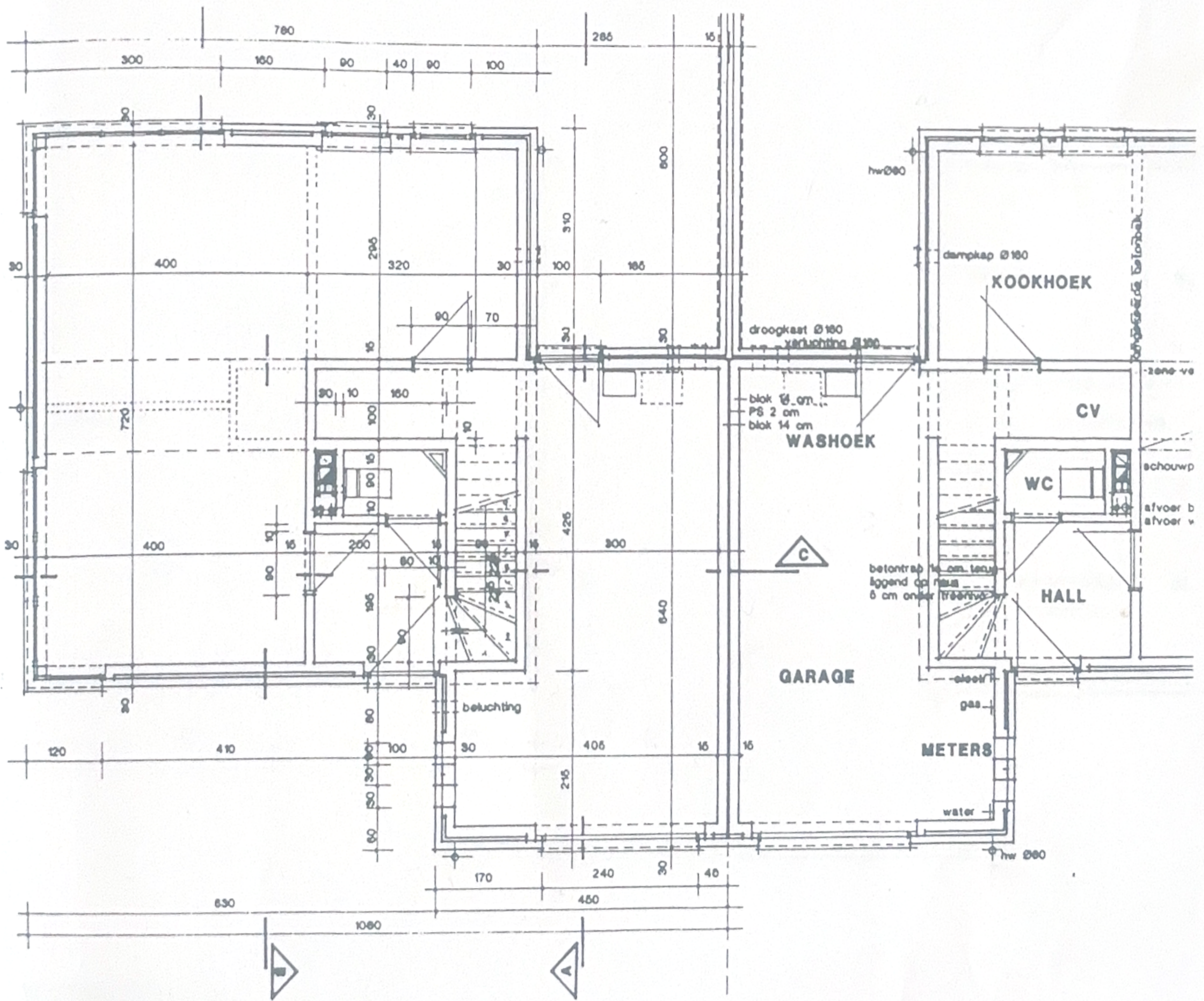
GRONDPLAN.
