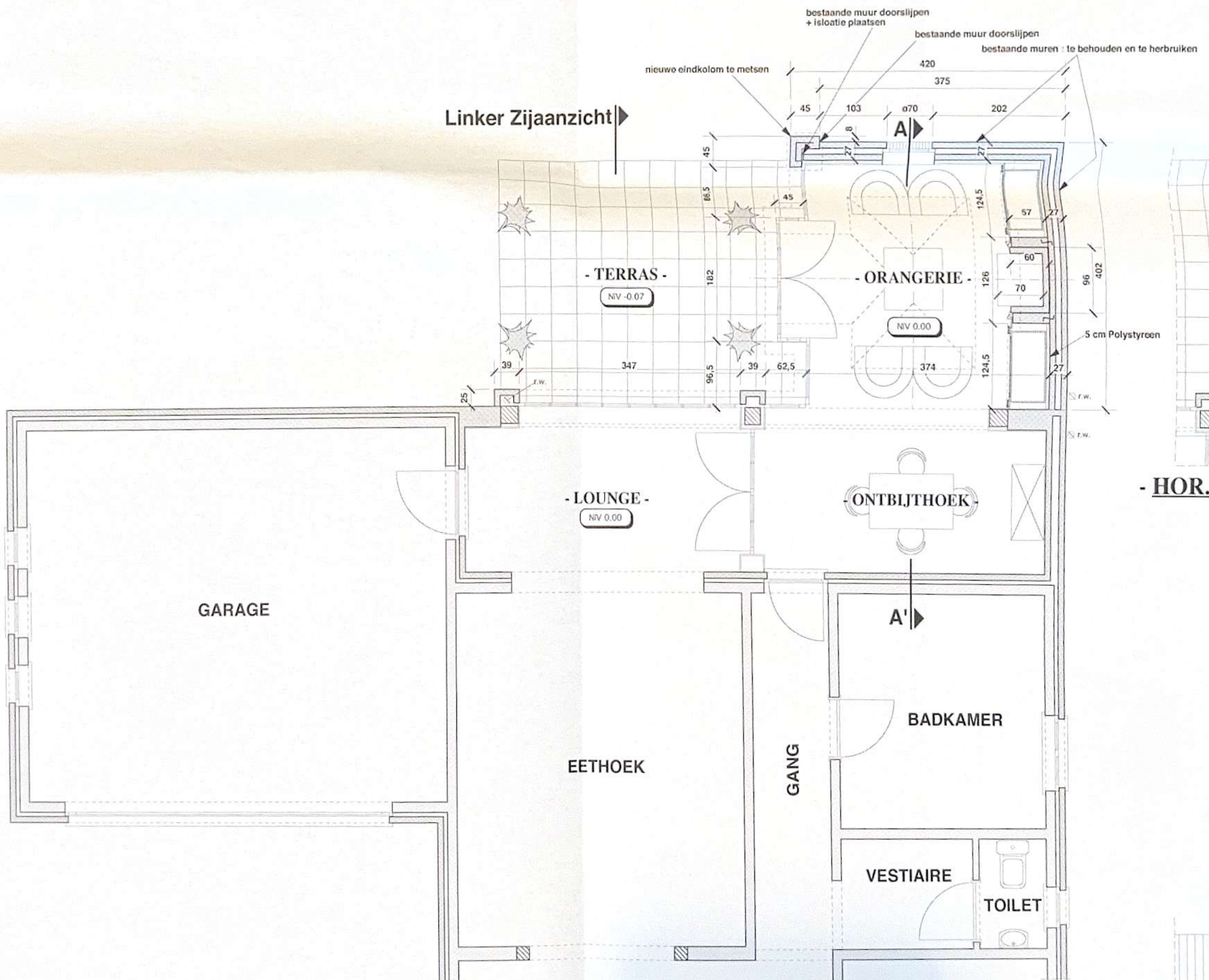
- NIEUW GRONDPLAN -
