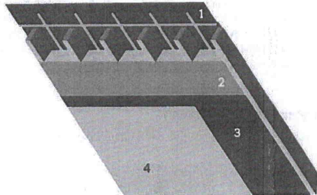
1. Onderdak | 2. Isolatie | 3. Dampscherm | 4. binnenafwerking
