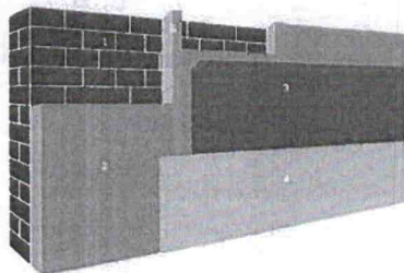
1. Buitenmuur | 2. Isolatie | 3. Vochtschermb | 4. Afwerkingslaag | 5. Stijl- en regelwerk (optioneel)
