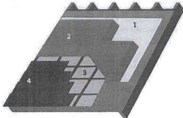
1. Dampscherm | 2. Isolatie | 3. Onderdak | 4. Dakbekleding
