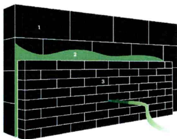
1. Dragende muur | 2. Ingeblazen isolatie | 3. Gevelsteen / gevelbekleding
