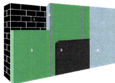
1. Buitengevel | 2. Isolatie | 3. Dampscherf | 4. Binnenafwerking | 5. Stijl- en regelwerk (optioneel)
