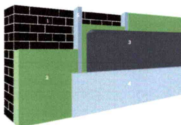
1. Buitenmuur | 2. Isolatie | 3. Vochtsschermb | 4. Afwerkingslaag | 5. Stijl- en regelwerk (optioneel)
