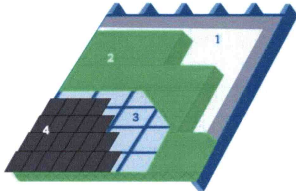
1. Dampscherm | 2. Isolatie | 3. Onderdak | 4. Dakbedekking
