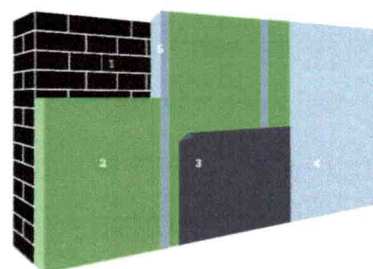
1. Buitengevel | 2. Isolatie | 3. Dampsschermb | 4. Binnenafwerking | 5. Stijl- en regelwerk (optioneel)
