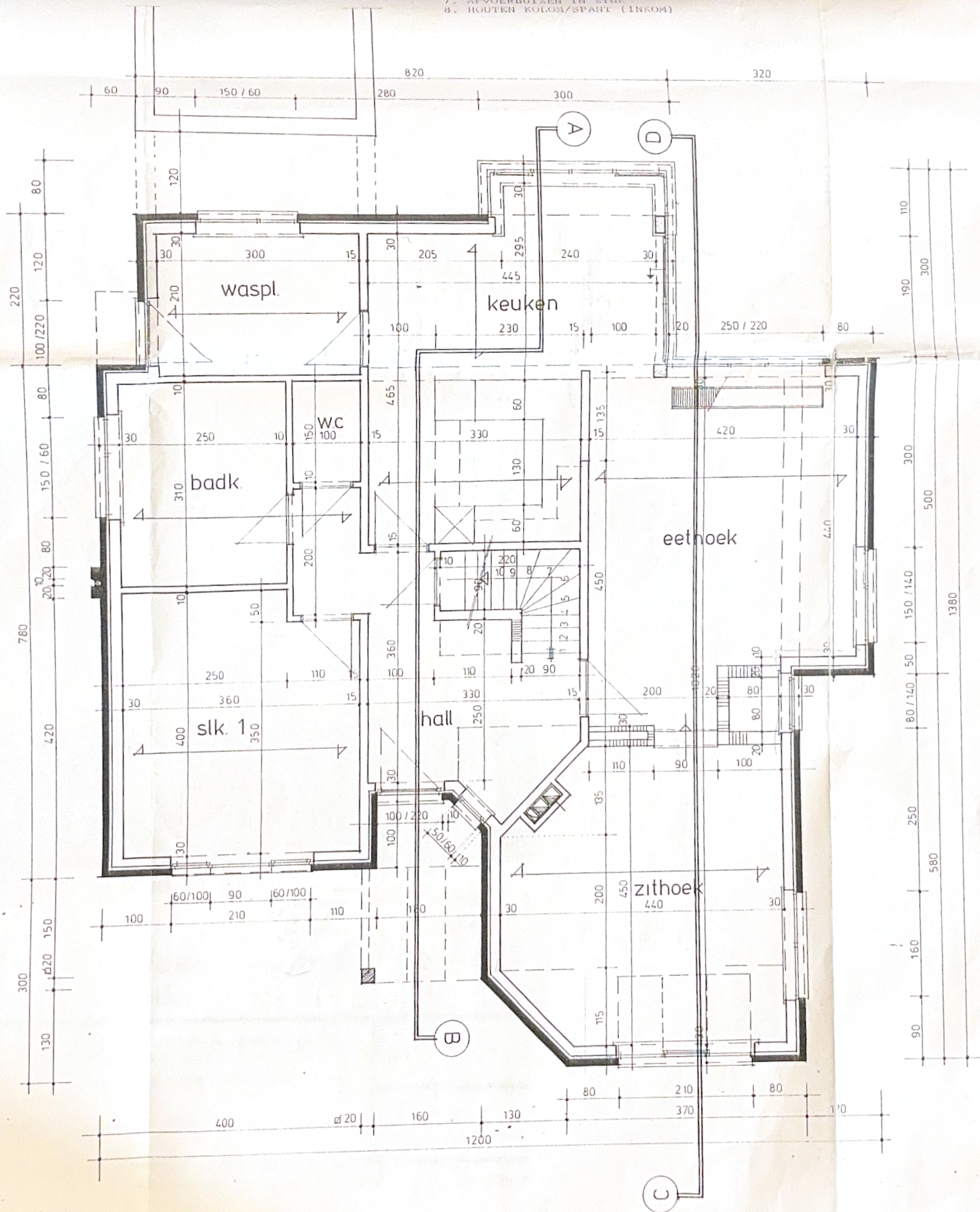
grondplan
