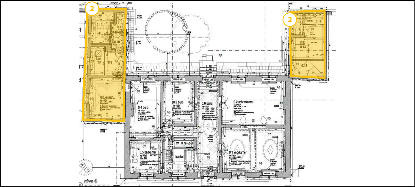
Legende van plan 1.6: Grondplan gelijkvloers 2
