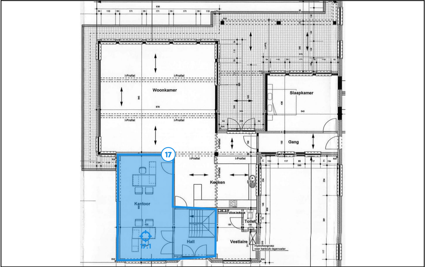
Legende van plan 1.5: GVL deel 3
